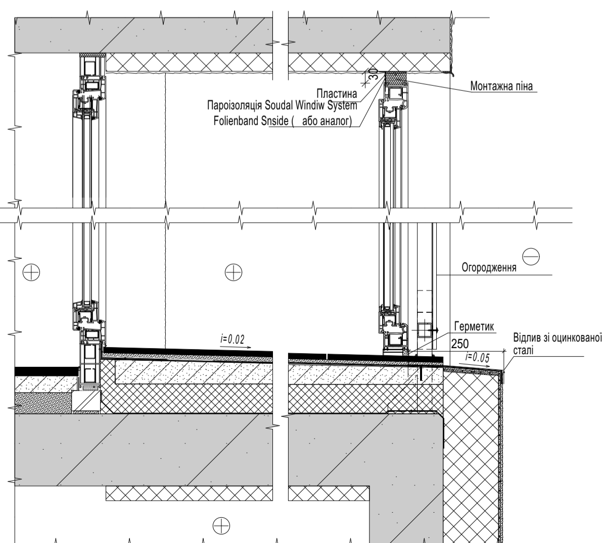
Розріз балкону улаштування скління на 2-му поверсі
