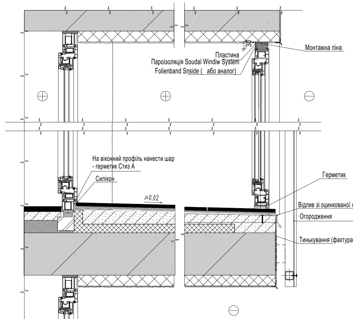
Розріз балкону улаштування скління на типовому поверсі
